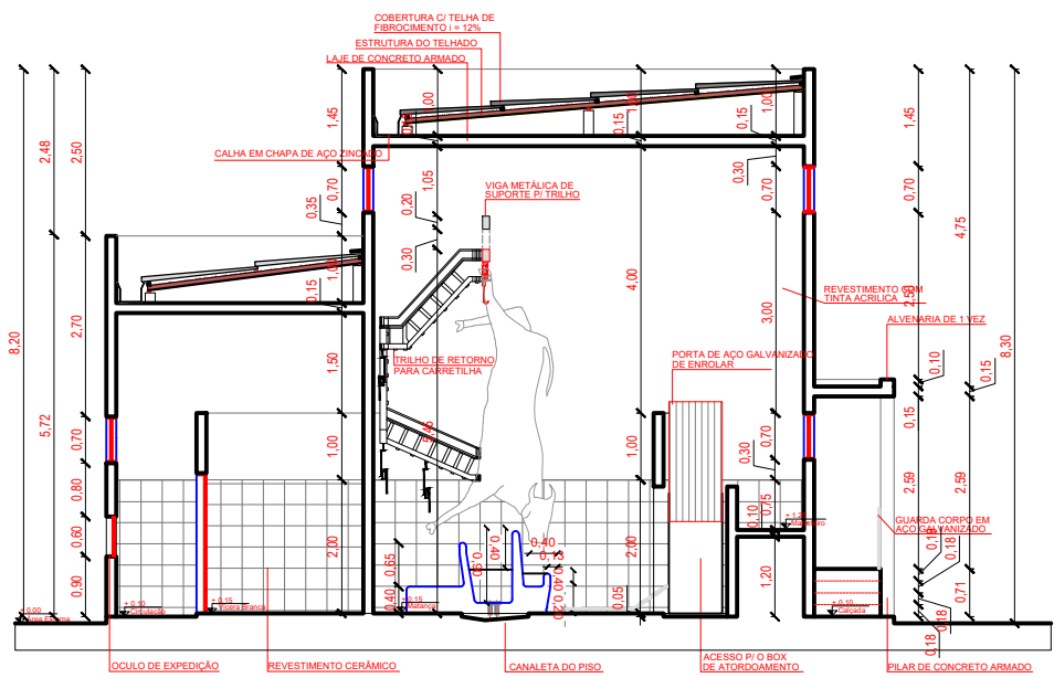
CORTE _ BB ESCALA 1/125
