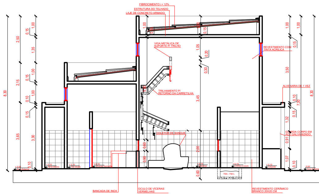
CORTE _ AA ESCALA 1/125
