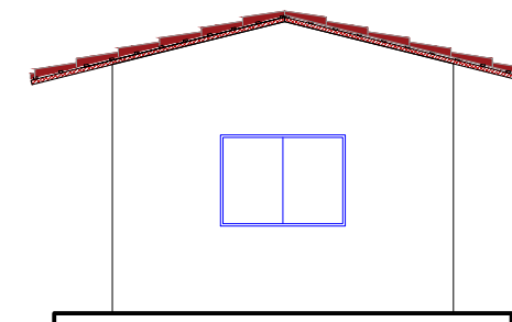
FACHADA LATERAL ESCALA 1/100
