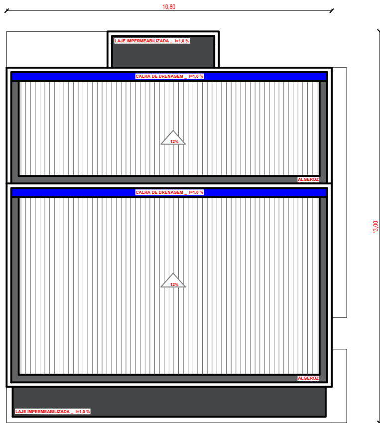
PLANTA DE COBERTA ESCALA 1/125
