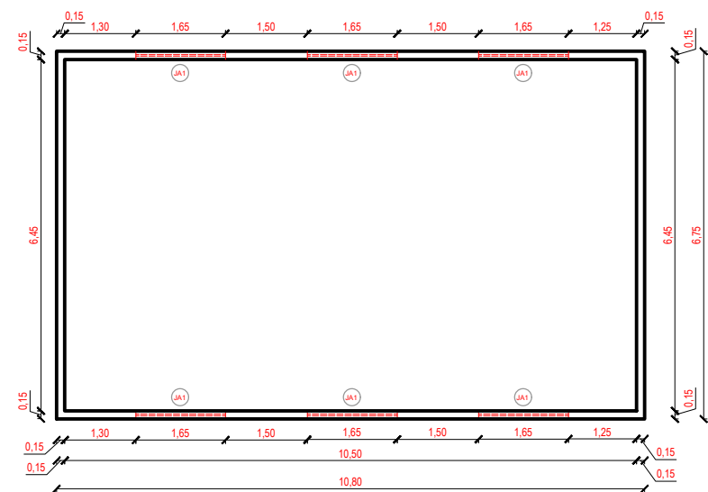
PLANTA BAIXA _ DETALHE ESQUADRIAS ELEVADAS ESCALA 1/125
